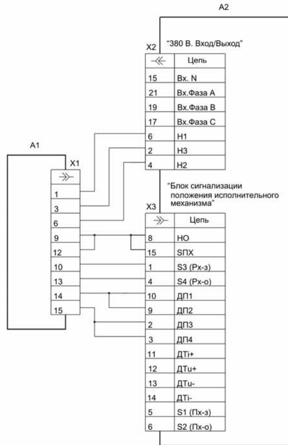
A1 - исполнительный электроприводной механизм МЭП2500 с блоком сигнализации положения БСПР-22; A2 - блок управления электроприводом БУЭП-2; X1 - розетка кабельная РП10-22ЛУ с кожухом НЩ0.364.005 ТУ; X2 - розетка кабельная РП10-22ЛУ с кожухом НЩ0.364.005 ТУ (входит в комплект поставки прибора); X3 - вилка кабельная ДВ-15М с кожухом (входит в комплект поставки прибора).
