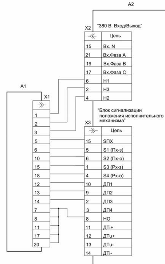
A1 - исполнительный электроприводной механизм МЭП6300 с блоком сигнализации положения БСПИ-10; A2 - блок управления электроприводом БУЭП-2; X1 - розетка кабельная РП10-22ЛУ с кожухом НЩ0.364.005 ТУ; X2 - розетка кабельная РП10-22ЛУ с кожухом НЩ0.364.005 ТУ (входит в комплект поставки прибора); X3 - вилка кабельная ДВ-15М с кожухом (входит в комплект поставки прибора).
