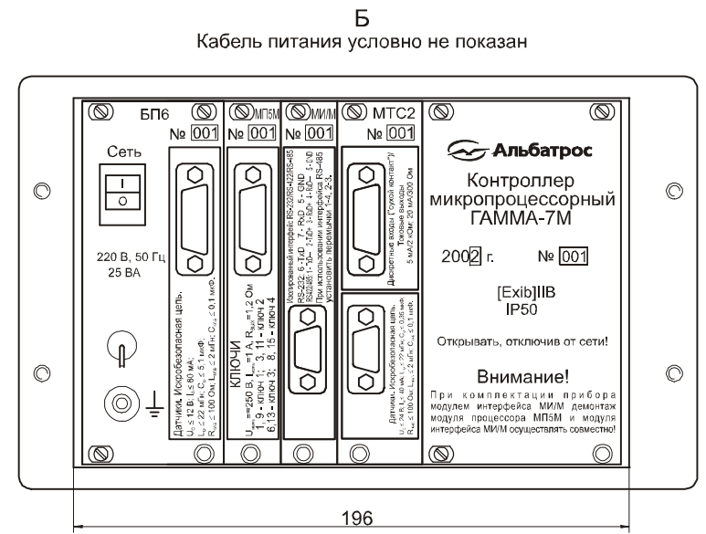
Рисунок 1 – Внешний вид и габаритные размеры прибора (на примере прибора исполнения 7)
