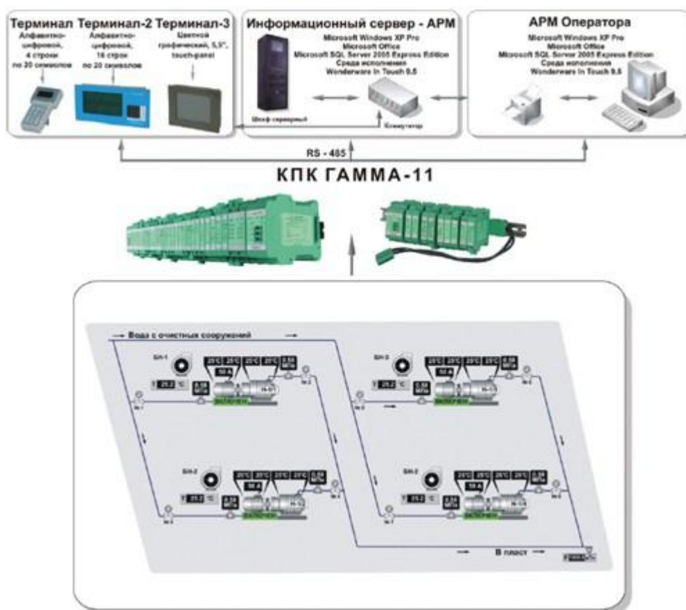
Рисунок 1 – Структурная схема автоматизированной системы контроля кустовой насосной станции
